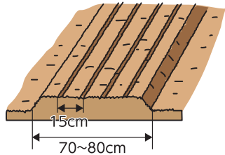
図3 トンネルの被覆
