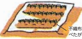
図4 間引き
